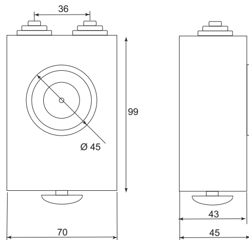
EMR150 Módulo electrónico selector de hoja
